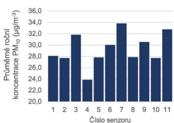
Obr. 11.15. Průměrné roční koncentrace \text{PM}_{10} v lokalitě Radvanice, 1.9.2019 – 31.8.2020, tabulka (vlevo) a graf (vpravo).
