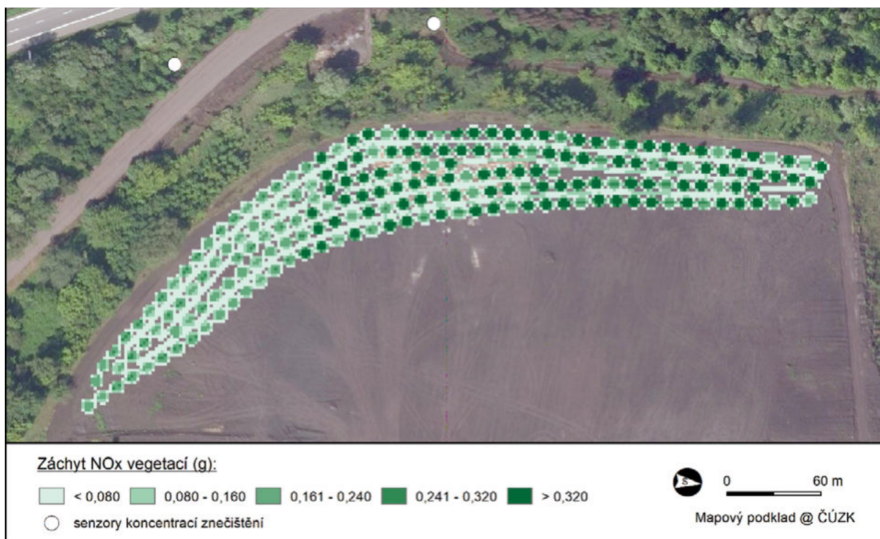
Obr. 15.8. Záchyt NO x (g) ve stavu po výsadbě navrhované vegetace v síti 1 x 1 m na lokalitě Bartovice. Modelováno pro období dvou měsíců (na konci vegetační sezony). V případě stavu před výsadbou se nepředpokládá vzhledem k absenci jakékoliv stávající zeleně významný záchyt znečištění.
