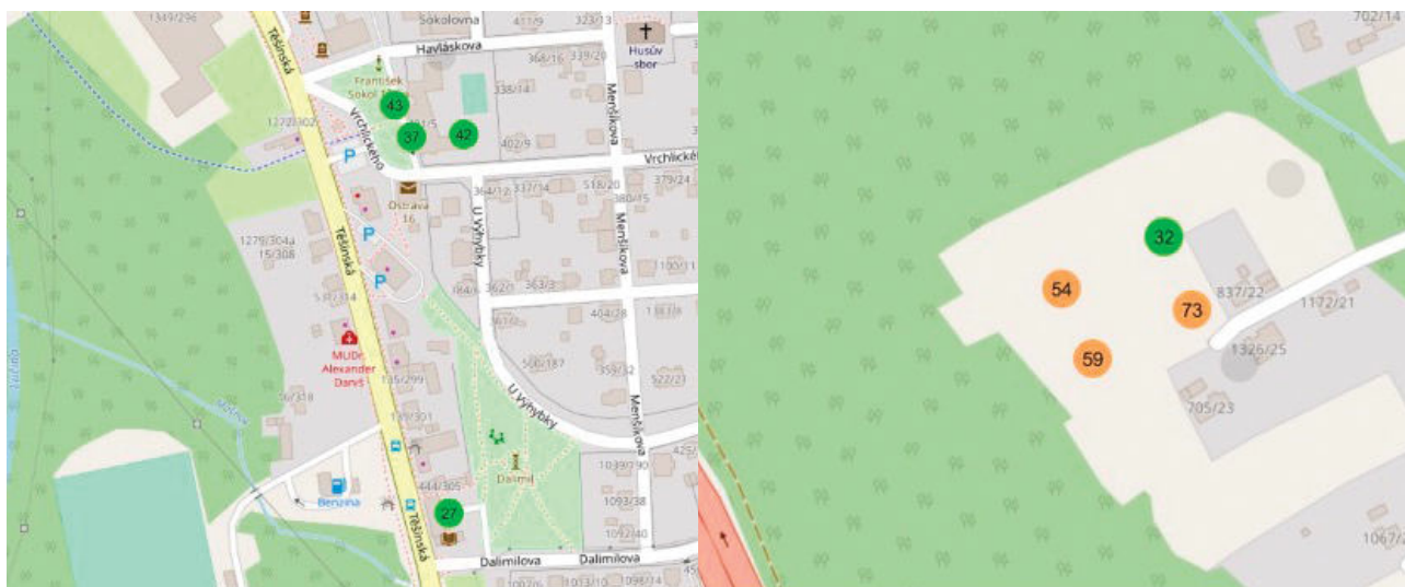
Obr. 11.9. Výřez mapy IIS – zobrazení naměřených koncentrací ( PM_{10} ).
